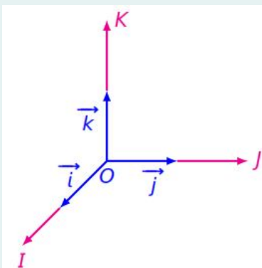
La base (\vec{i}; \vec{j}; \vec{k}) est directe
